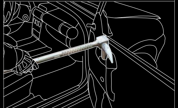
Openingsopties bij de binnendeur
