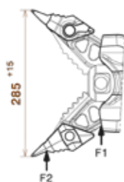
Standaard tip Onderdeelnr. 3867323
